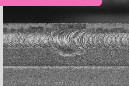
局所的な溶接ムラ
